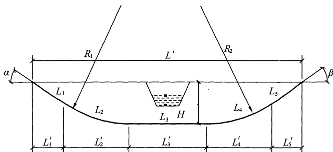
图 A. 0. 1 钻孔轨迹
