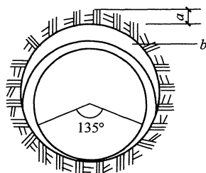
图 1 超挖示意图
